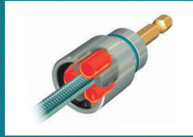
Fixando porcas no parafuso em locais altos
