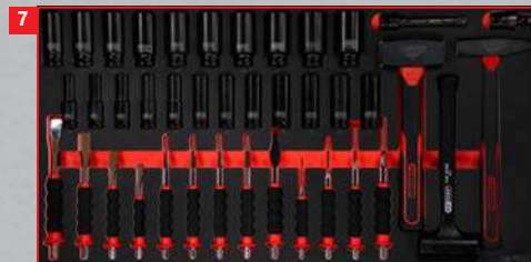
Kit de martelo, escopro e pontas de chave de caixa de impacto
